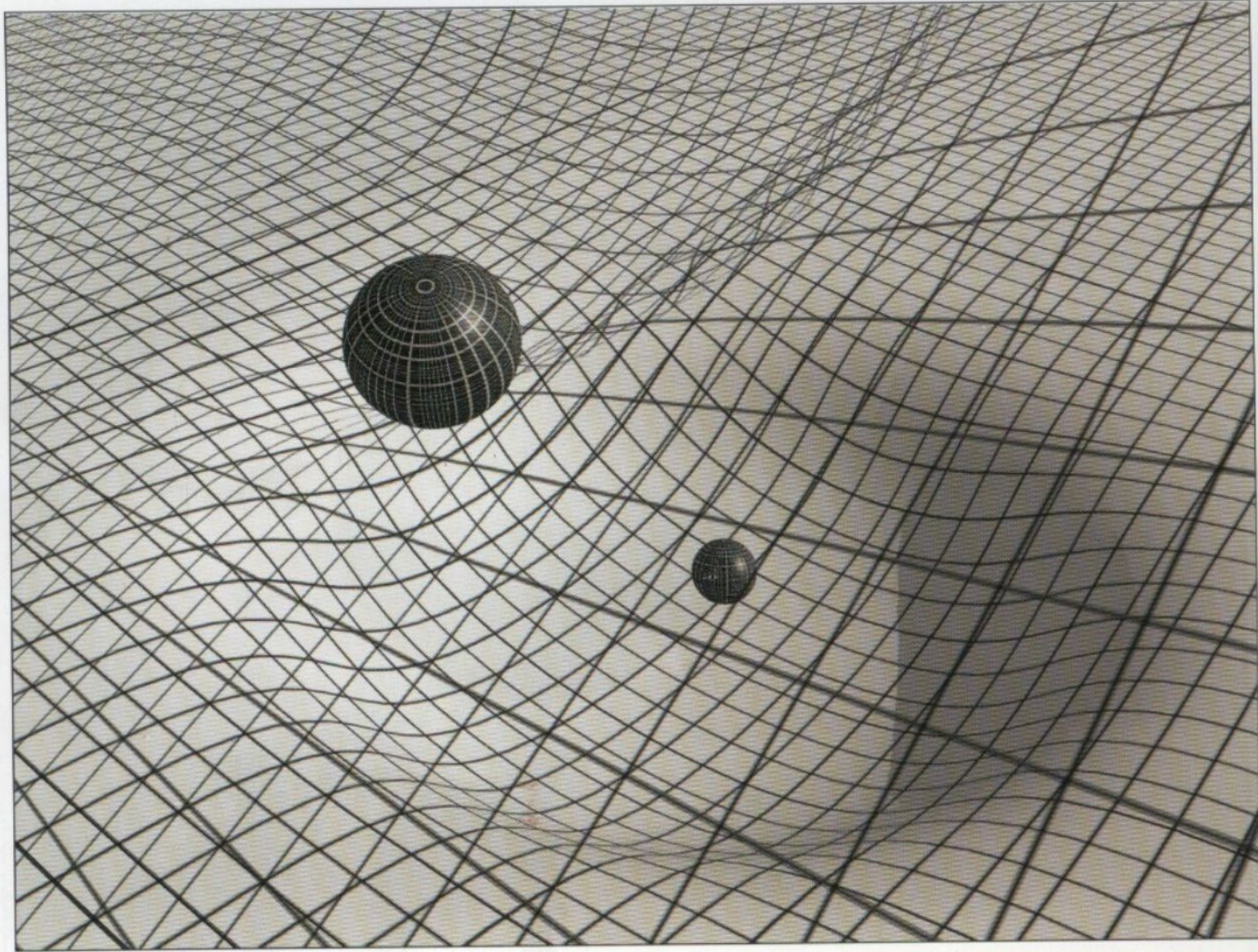
(ŞEKİL 1.12) UZAY-ZAMAN EĞRİLERİ
