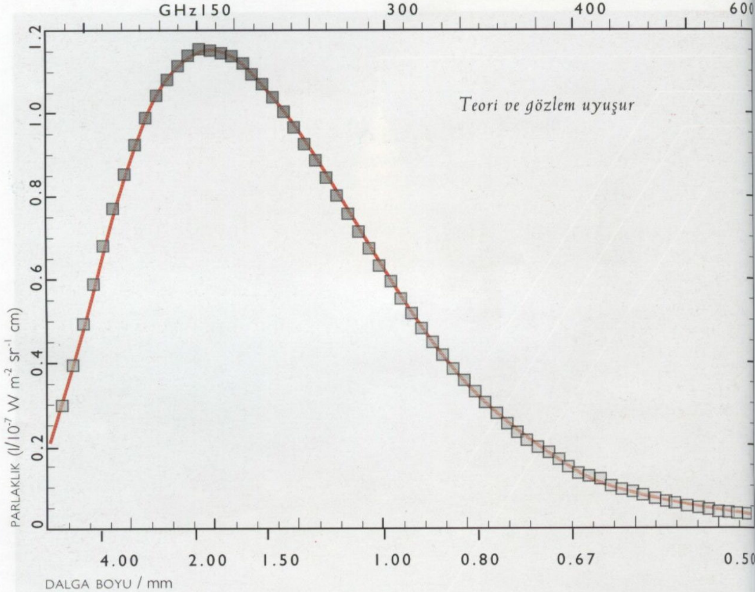
(ŞEKİL 2.6) MİKRODALGADA FON TAYFININ ÖLÇÜMÜ
