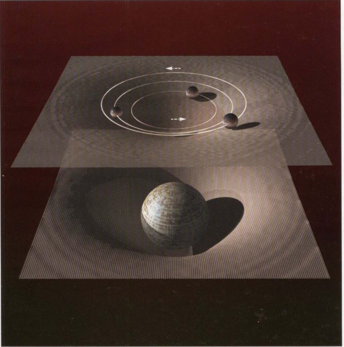
(ŞEKİL 7.12) Zar dünyası senaryosunda, kütle çekimin ek boyutlara nüfuz etmesi nedeniyle, gezegenler bir gölge zar üzerindeki karanlık bir kütle etrafında dönebilir.
