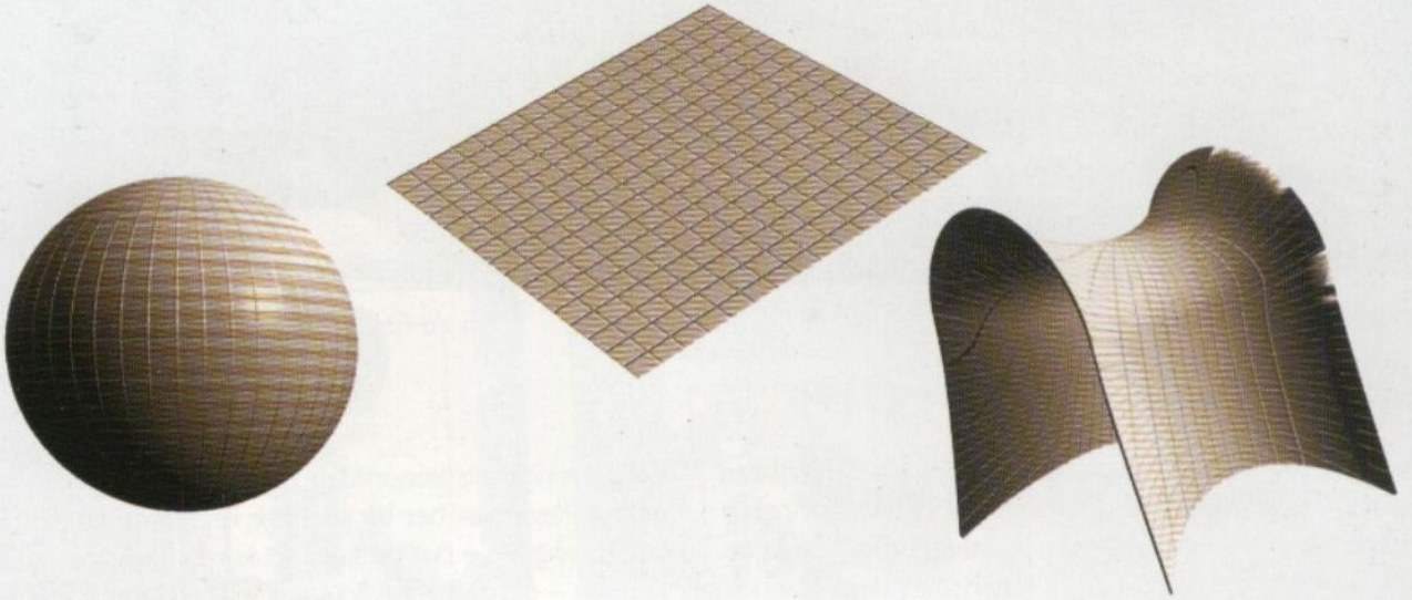
(ŞEKİL 3.9) EVRENİN GEÇMİŞLERİ
