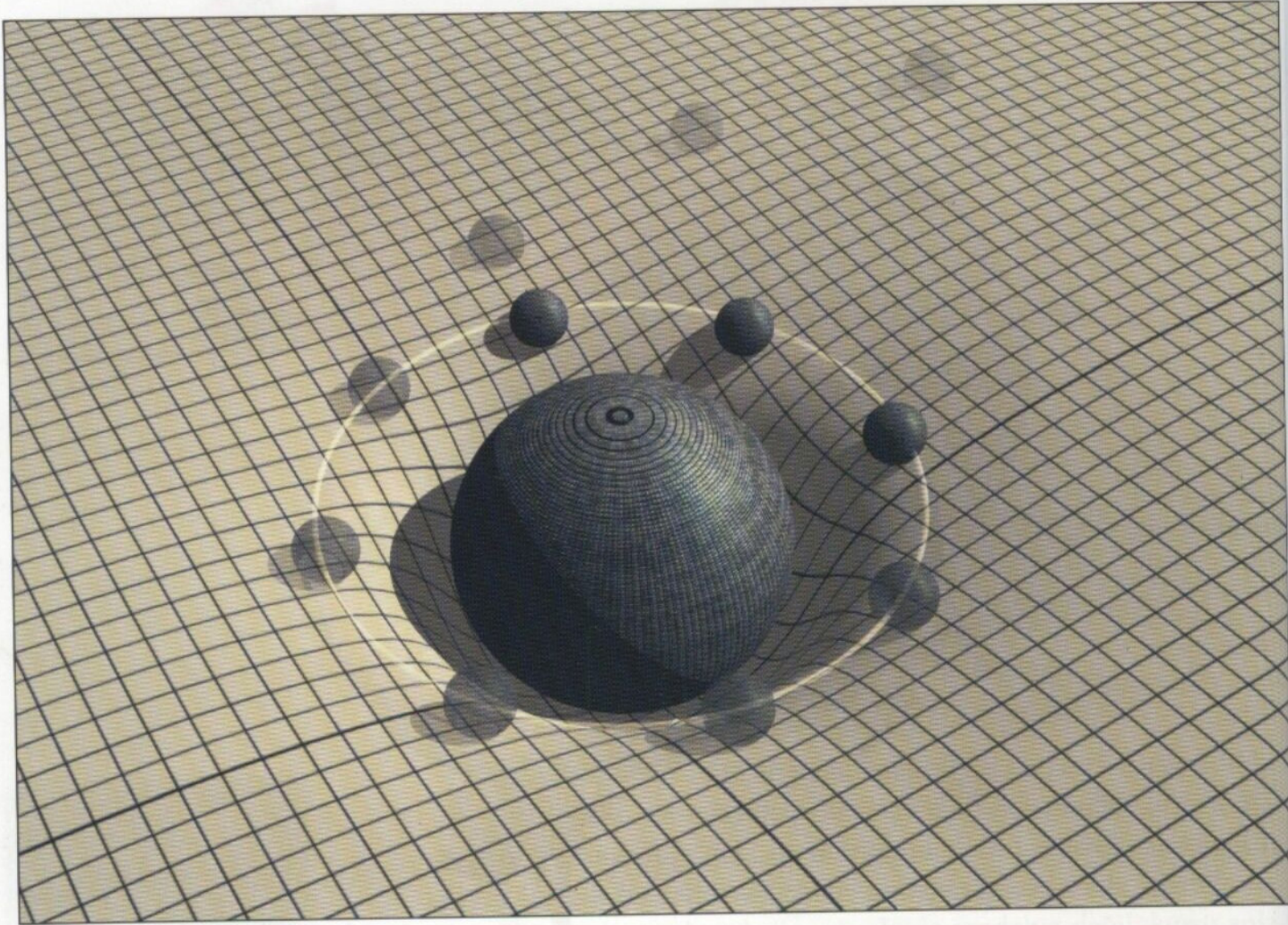
(ŞEKİL 2.4) KAUÇUK YAPRAK ÖRNEKSEMESİ
