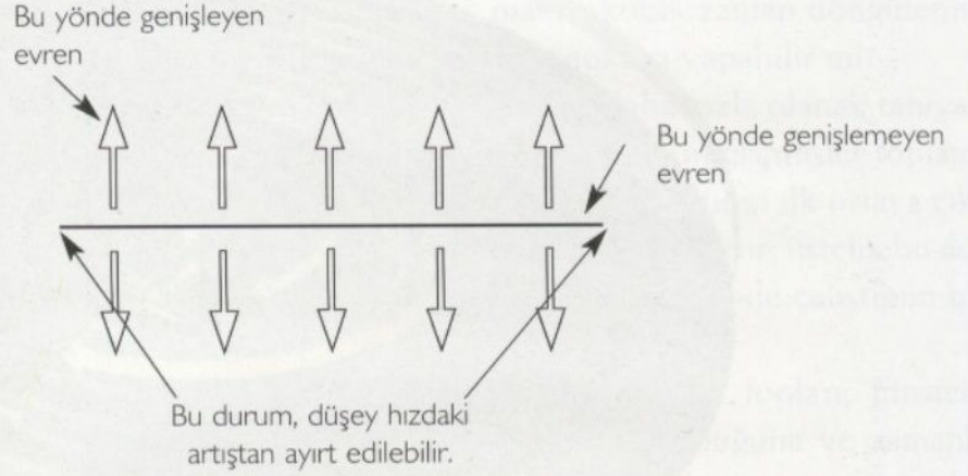
(ŞEKİL 5.18) ZAMAN-BENZERİ KAPALI EĞRİLERE SAHİP FON
