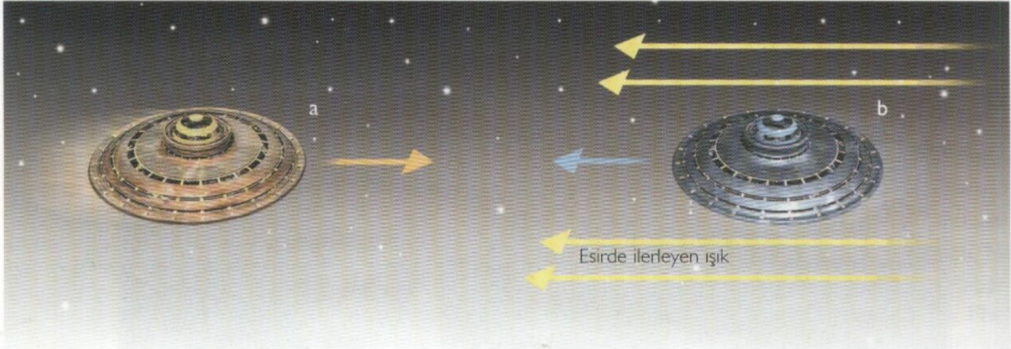
(ŞEKİL 1.1, yukarıda) SABİT ESİR TEORİSİ
