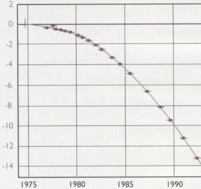
PSR 1913 + 16 ikili pulsarının 1975'ten bu yana grafiği
