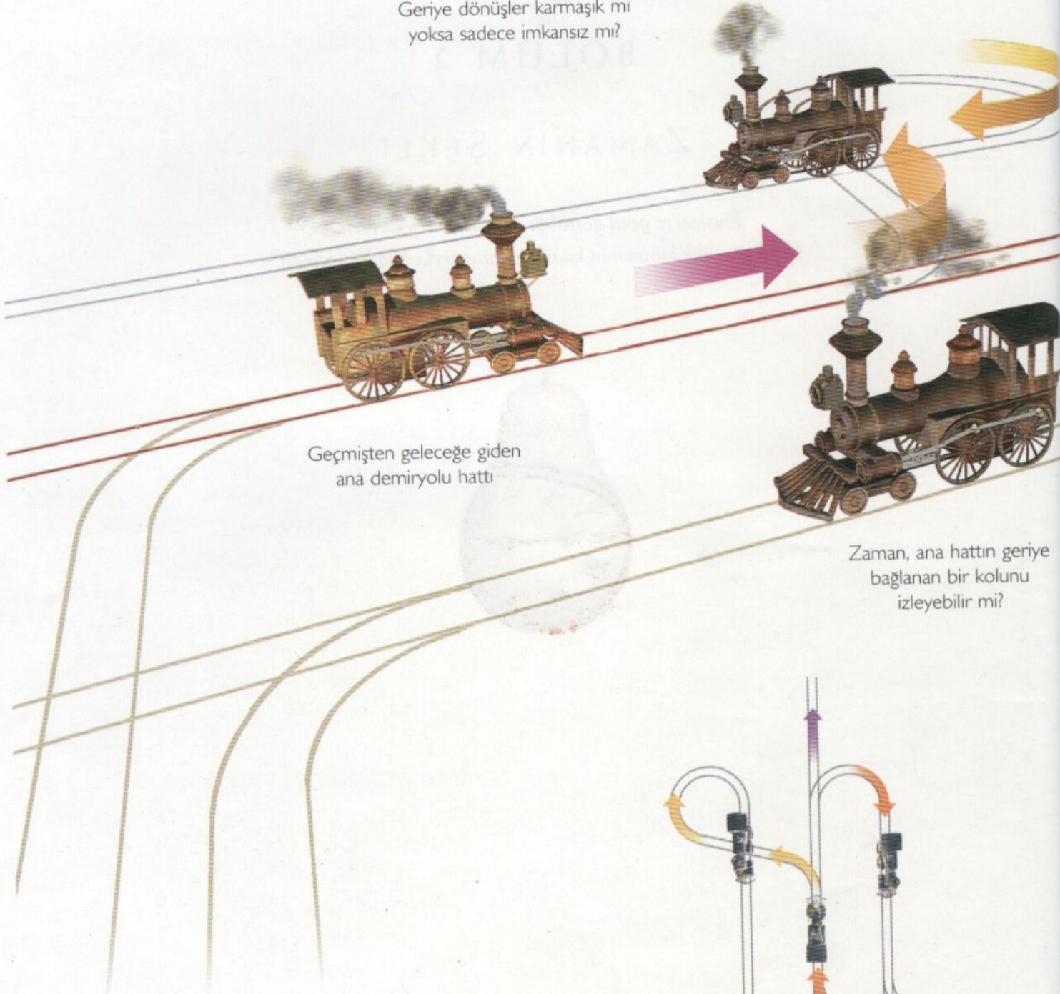
(ŞEKİL 2.1) ZAMANIN BİR DEMİRYOLU ŞEKLİNDEKİ MODELİ
