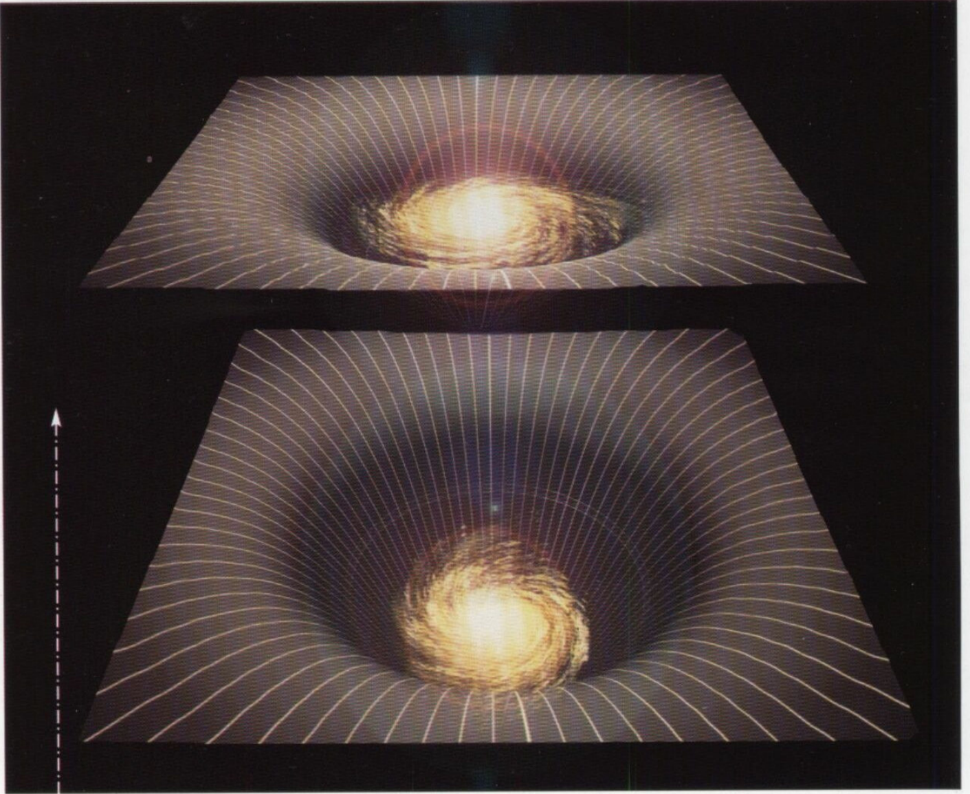
Zarlar arasında uzanan, ek boyutların bulunduğu ıssız bölge.
