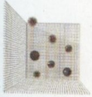
Parçacığın konumunun belirsizliği
