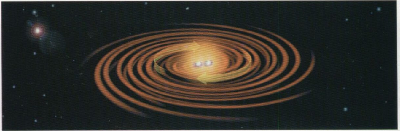
Birbirine yaklaşıarak spiral çizen yoğun iki nötron yıldızı
