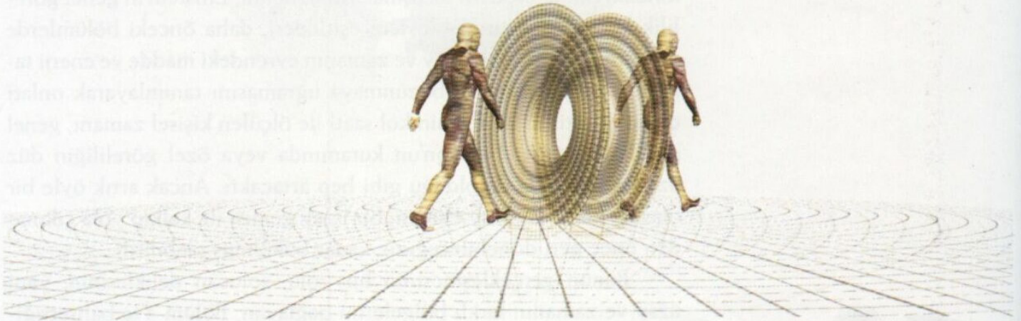
(ŞEKİL 5.2) İKİZLER PARADOKSUNUN İKİNCİ BİR ÇEŞİDİ
